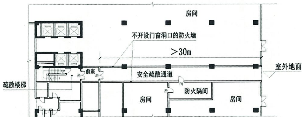
附图62: 安全疏散通道设置
